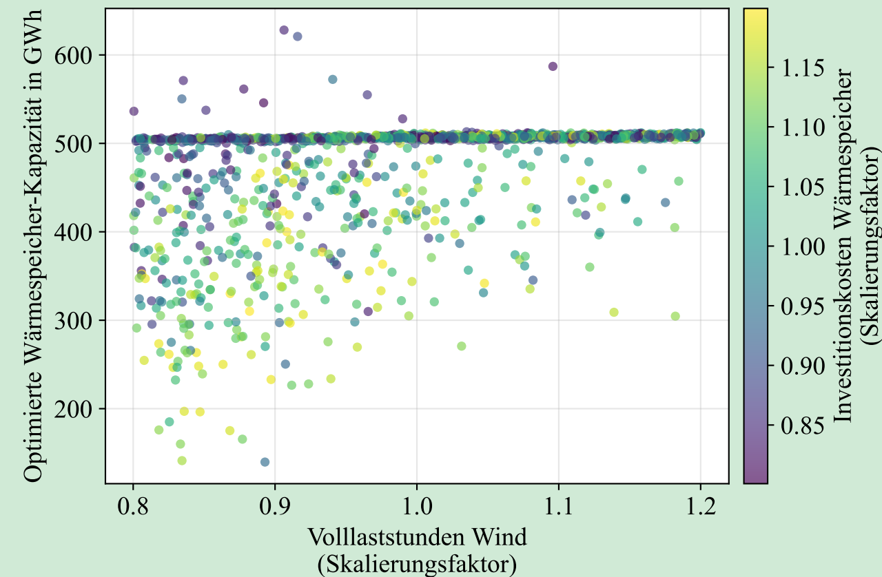
4. Parameterinteraktion Volllaststunden Wind vs. Investitionskosten Wärmespeicher
