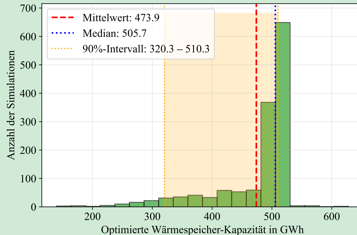
3. Unsicherheit Optimierte Wärmespeicher-Kapazität aus 1,400 Simulationen
