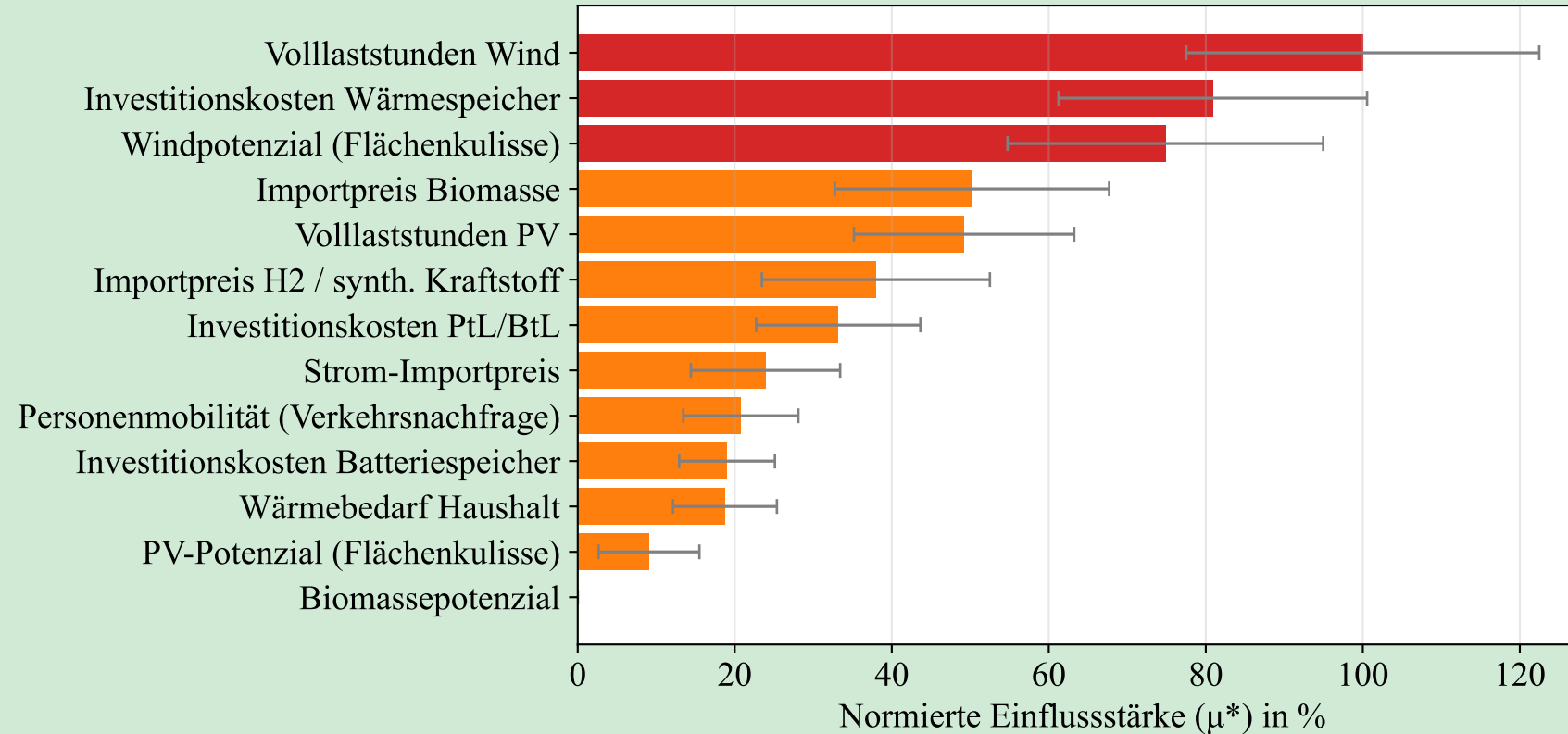
3. Unsicherheit Optimierte Wärmespeicher-Kapazität aus 1,400 Simulationen
